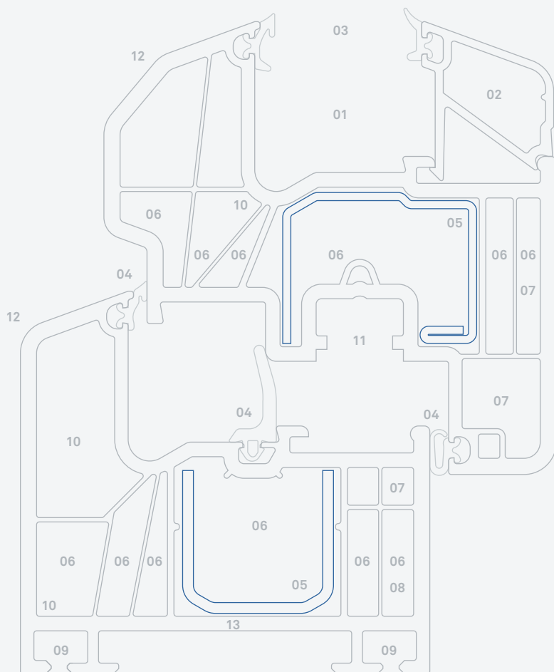
Prestige s předsazeným hranatým křídlem I 76.6 C4 Těsnění uprostřed (MD)
