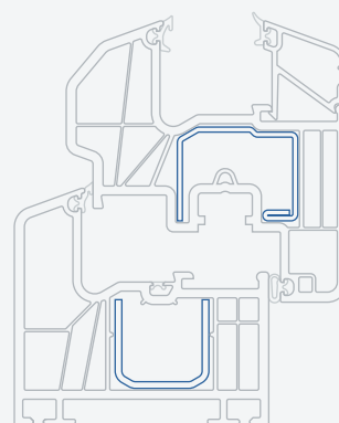
Prestige s předsazeným hranatým křídlem I 76.6 C4 Těsnění na dorazu (AD)
